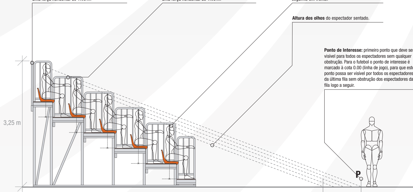
Módulo de Cadeiras em corte
