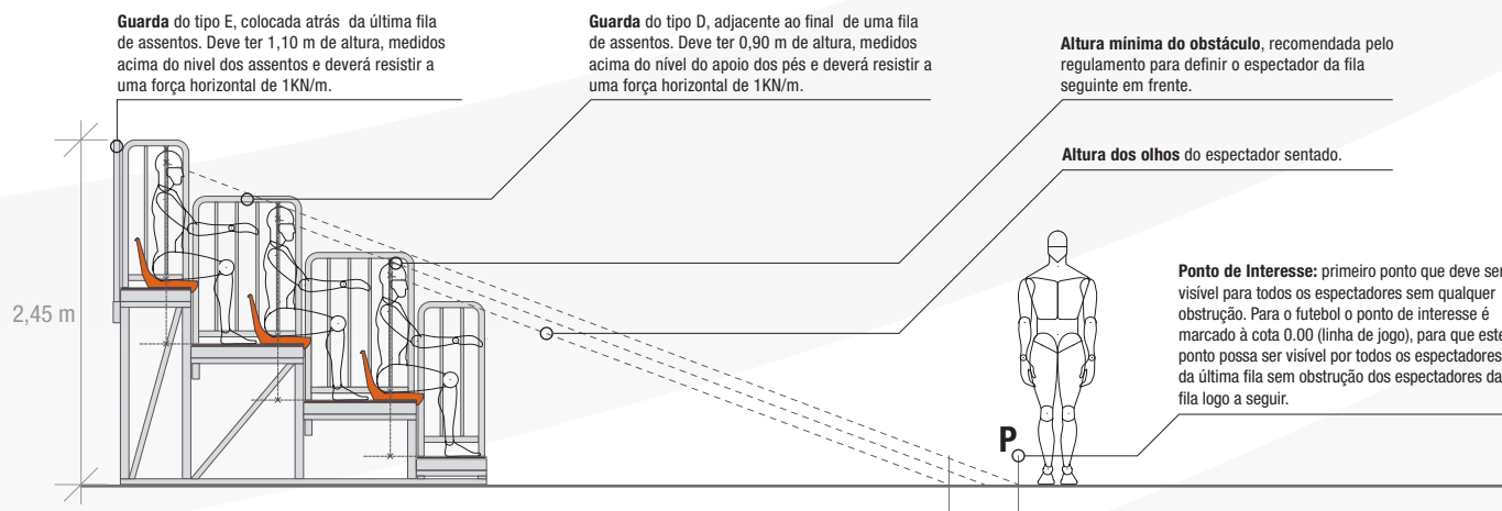
Módulo de Cadeiras em corte
